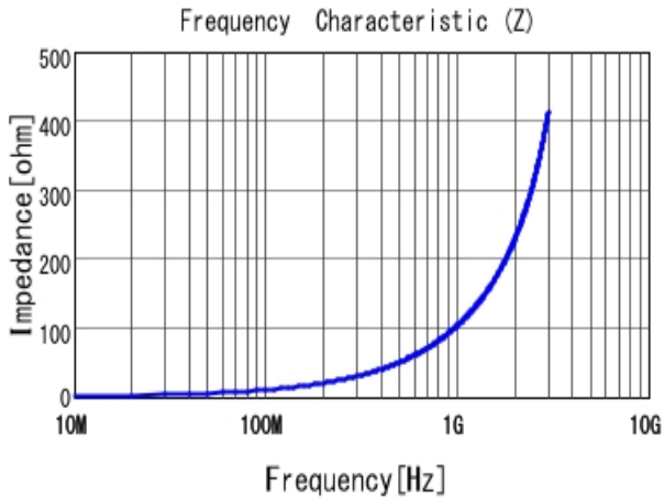
■ LQW18AN16NG00 |Z|
