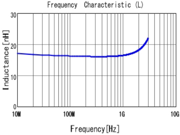
■ LQW18AN16NG00 L
