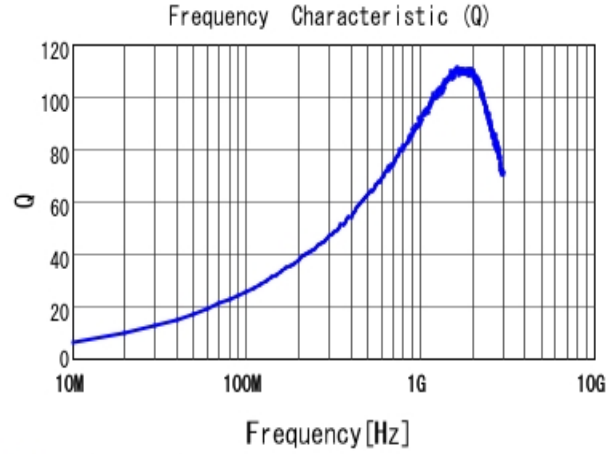
■ LQW18AN16NG00 Q
