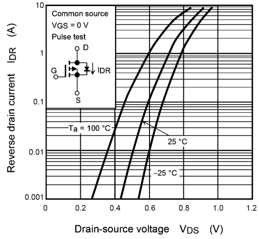
Fig. 8.8 I_{DR} - V_{DS}
