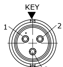
WIRING END W6282-3SG-P-3XX
