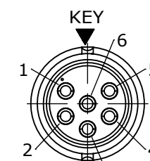
WIRING END W6282-6SG-P-3XX
