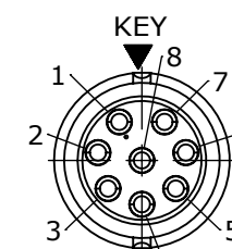
WIRING END W6282-8SG-P-3XX
