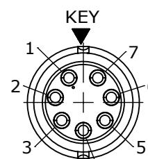
WIRING END W6282-7SG-P-3XX
