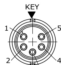
WIRING END W6282-5SG-P-3XX
