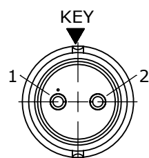
WIRING END W6282-2SG-P-3XX
