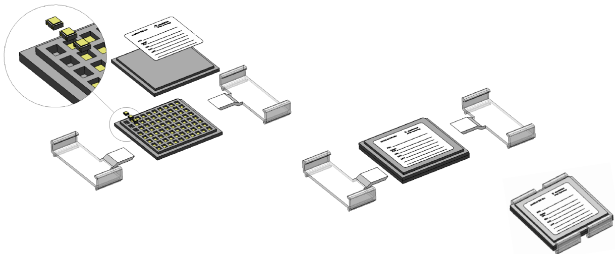
Waffle Pack
