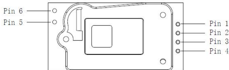
图 3.ACD10 引脚图
