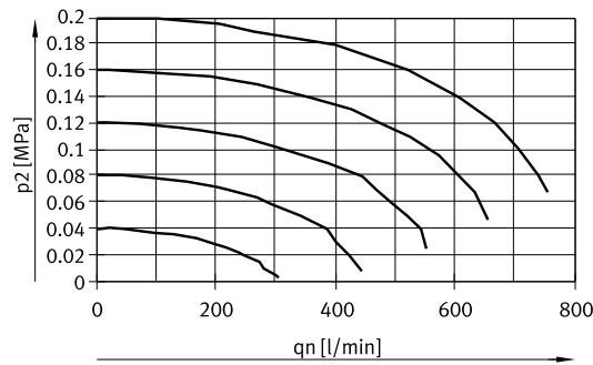
Fig. 5 VPPE-3-1-1/8-2-... p1 = 0.4 MPa
