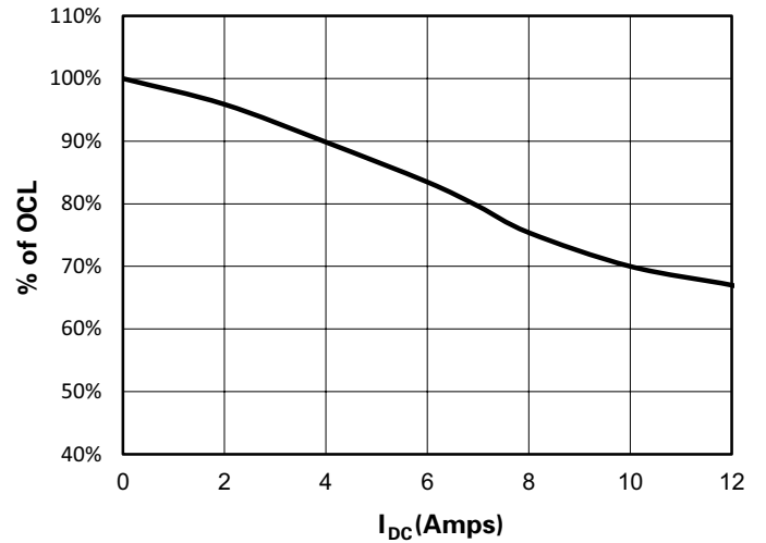
HCM0503-1R5-R
