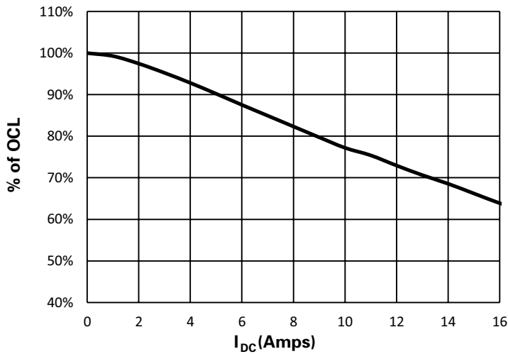
HCM0503-1R0-R
