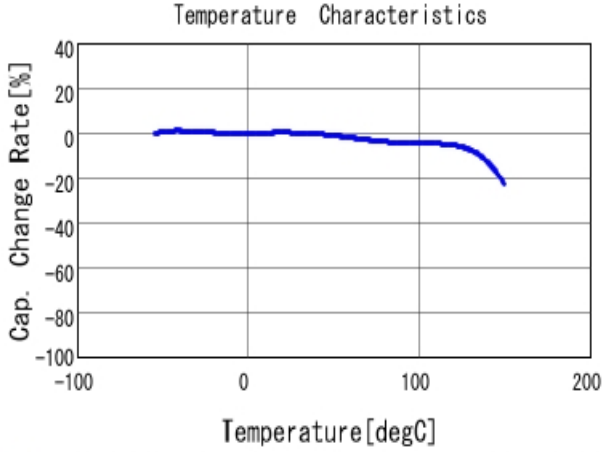
GCM188L81H104KA57 C-Temp. capchange, DCO. 0V, AC1.0V rm
