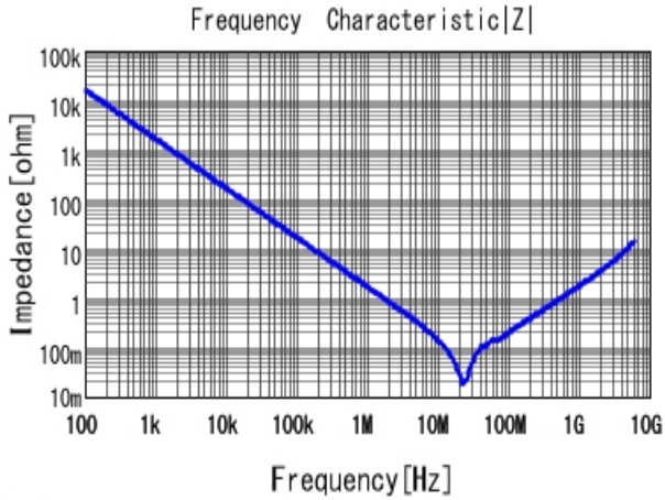
GCM188L81H104KA57 |Z| DC0V, 25degC
