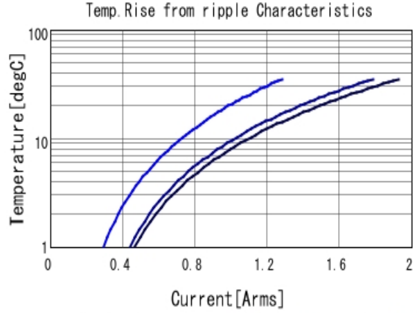
GCM188L81H104KA57 Temp. rise ■ 400kHz ■ 800kHz ■ 1MHz
