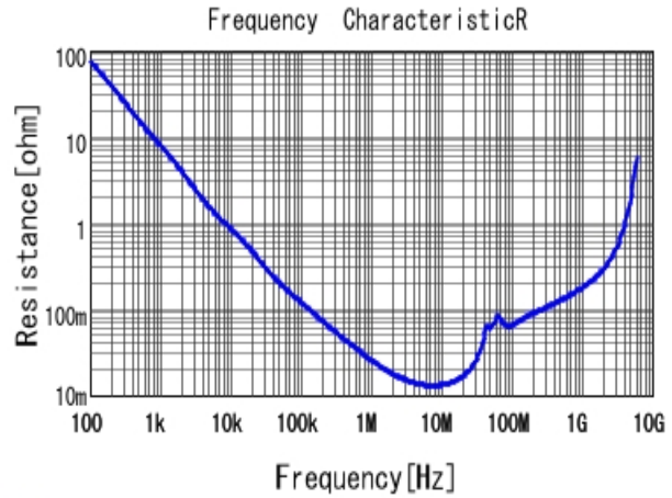
GCM188L81H104KA57 R DC0V, 25degC
