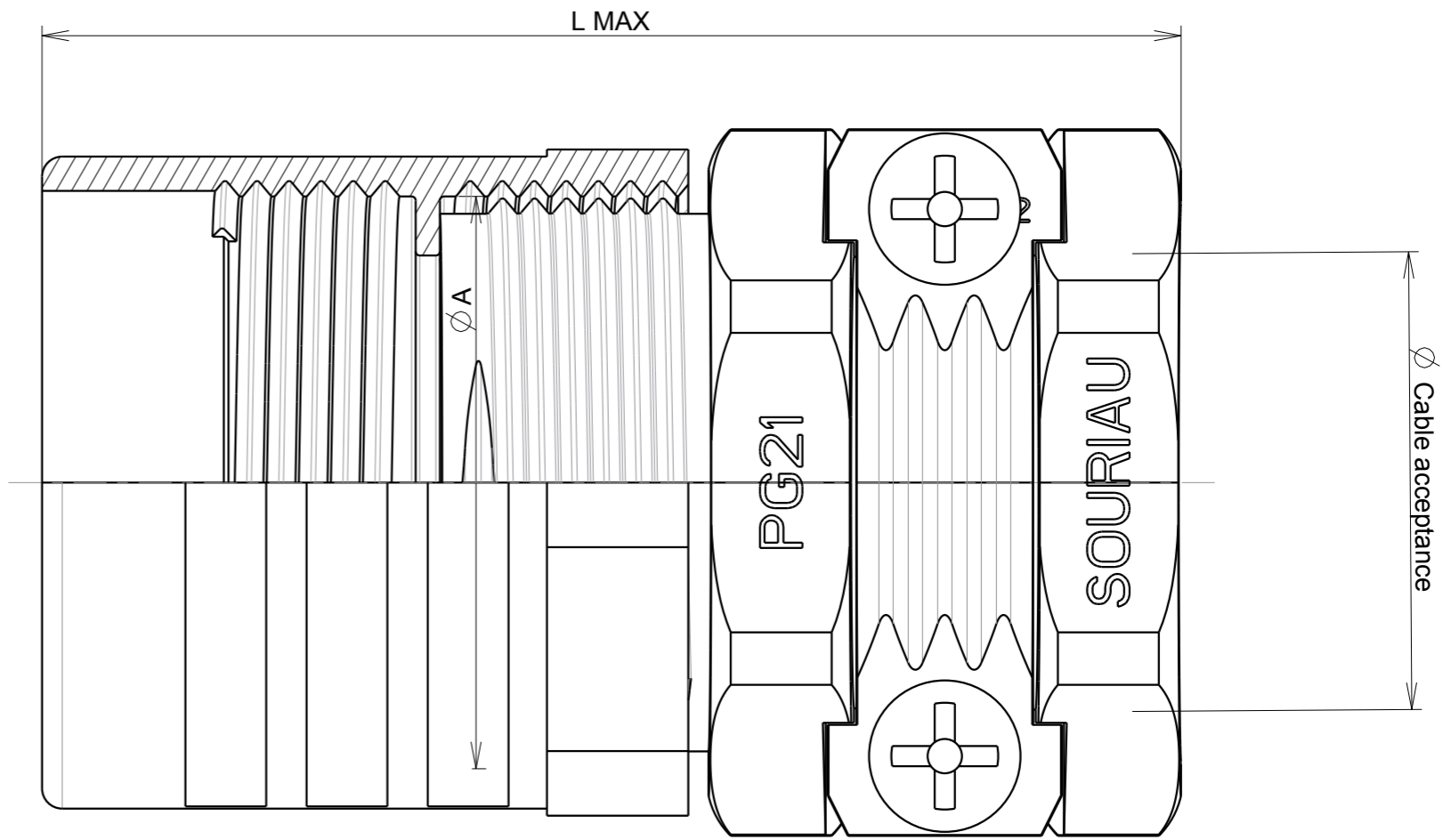
COUPE B-B
