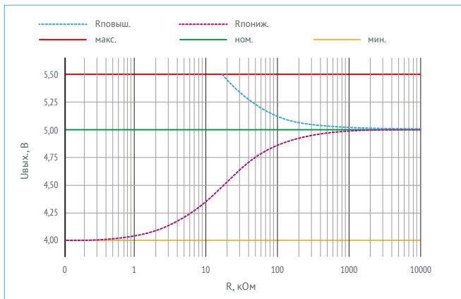
Рис. 6. График зависимости для VDRW100N05.
