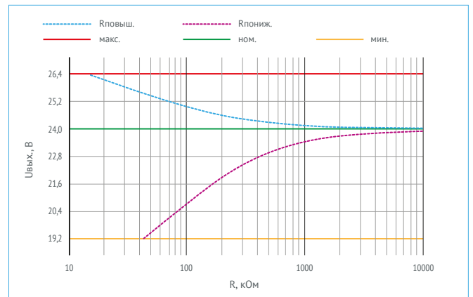
Рис. 9. График зависимости для VDRW100N24.
