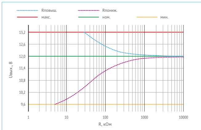
Рис. 7. График зависимости для VDRW100N12.
