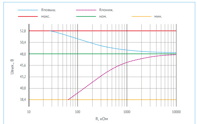
Рис. 11. График зависимости для VDRW100N48.
