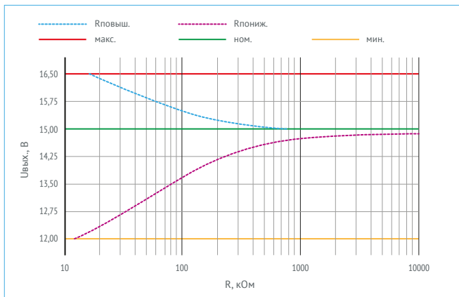
Рис. 8. График зависимости для VDRW100N15.
