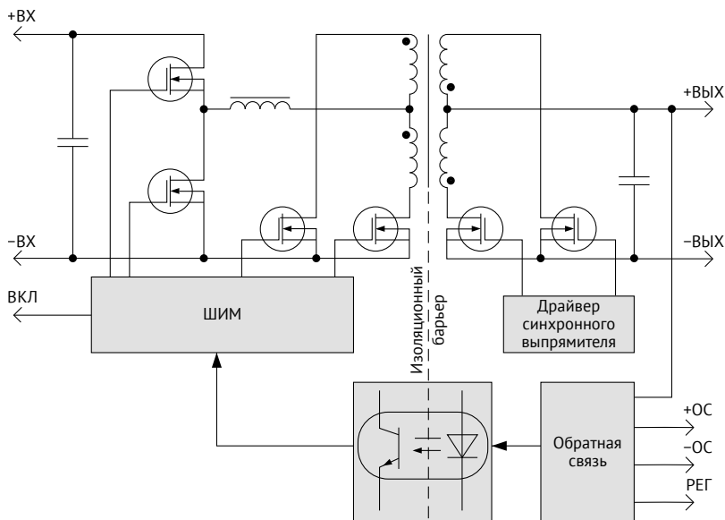
Рис. 1. Топология VDRW100.
