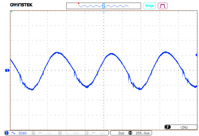
Рис. 27. Пульсации U_{\text{вых.ном}} .
