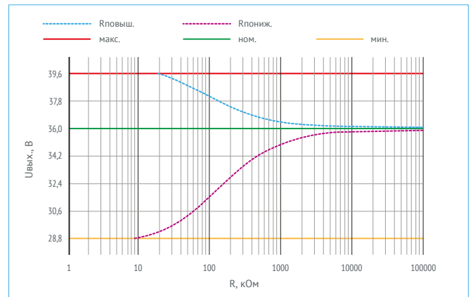
Рис. 10. График зависимости для VDRW100N36.
