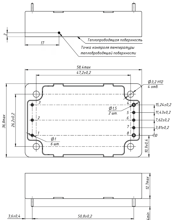
Рис. 30. Исполнение 1/4 Brick.
