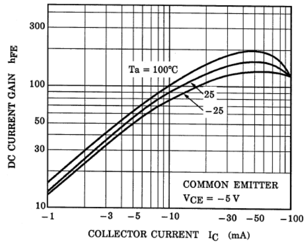
Fig. 10.14 RN2102 h_{FE}-I_C
