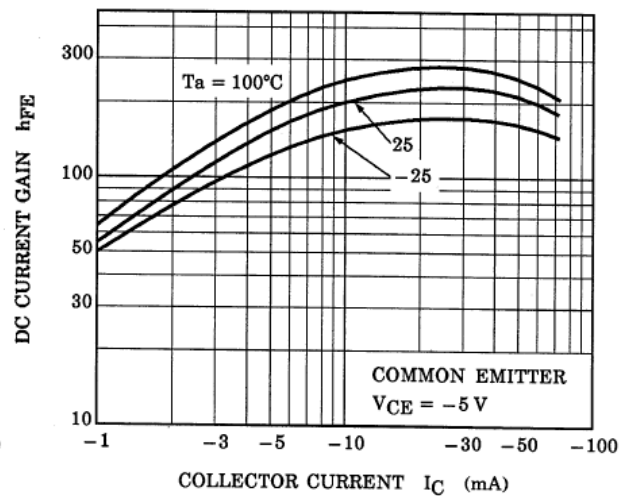
Fig. 10.16 RN2104 h_{FE}-I_C
