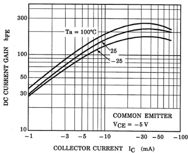
Fig. 10.15 RN2103 h_{FE}-I_C
