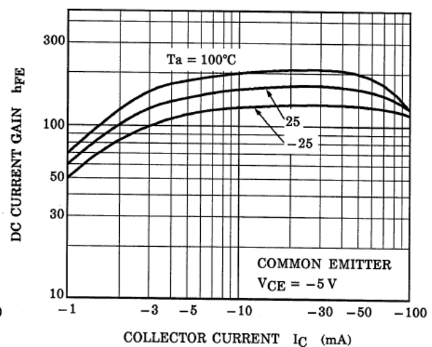
Fig. 10.18 RN2106 h_{FE}-I_C
