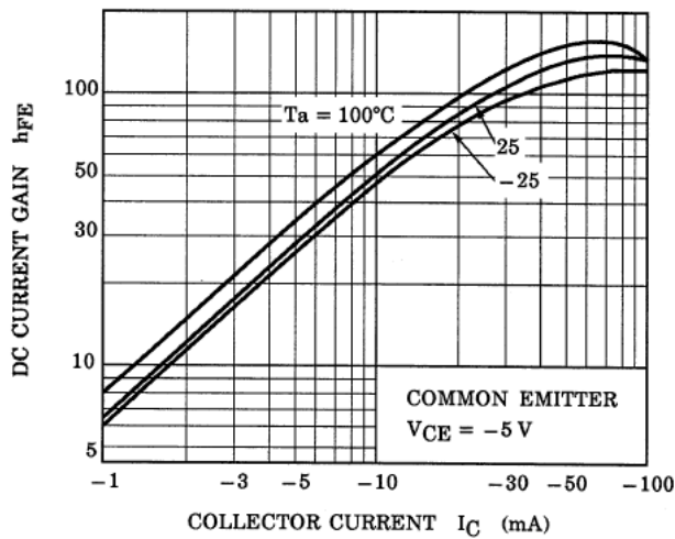
Fig. 10.13 RN2101 h_{FE}-I_C
