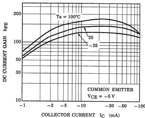
Fig. 10.17 RN2105 h_{FE}-I_C
