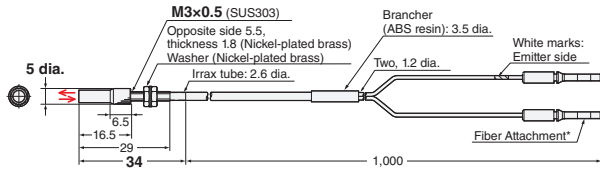
27-A E32-C41 1M (No Cutting) + E39-F3A-5
