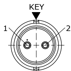
WIRING END W6280-2SG-P-5XX
