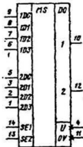
Условное графическое обозначение К134КП9
