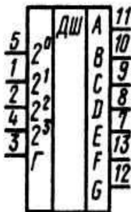
Условное графическое обозначение К514ИД1, КР514ИД1
