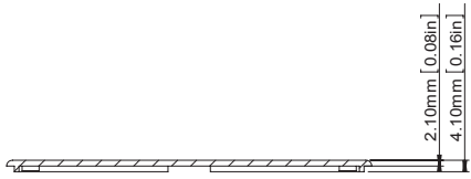
SECTION B-B SCALE 2 : 3
