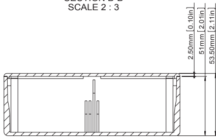
SECTION B-B SCALE 2 : 3
