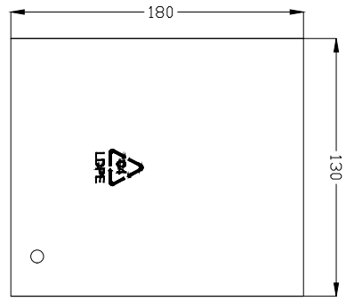
PE BAG:L180*W130*TO.05mm
