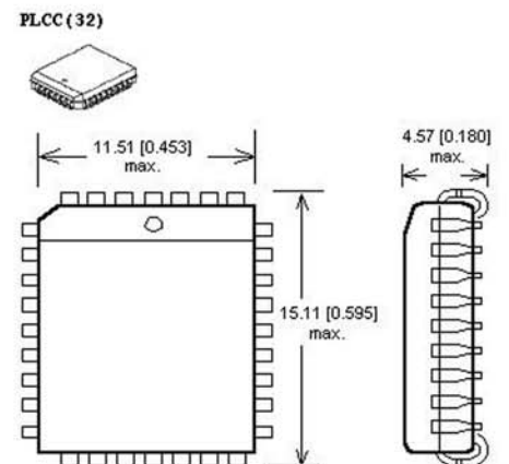
Package PLCC32 :
