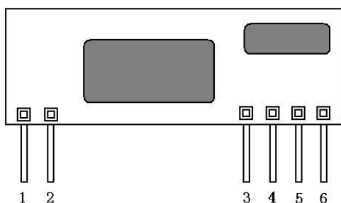
1:ANT 2:GND 3:VDD 4:DATA 5:DATA 6:GND
