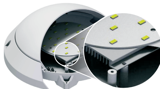
Алюминиевый радиатор
