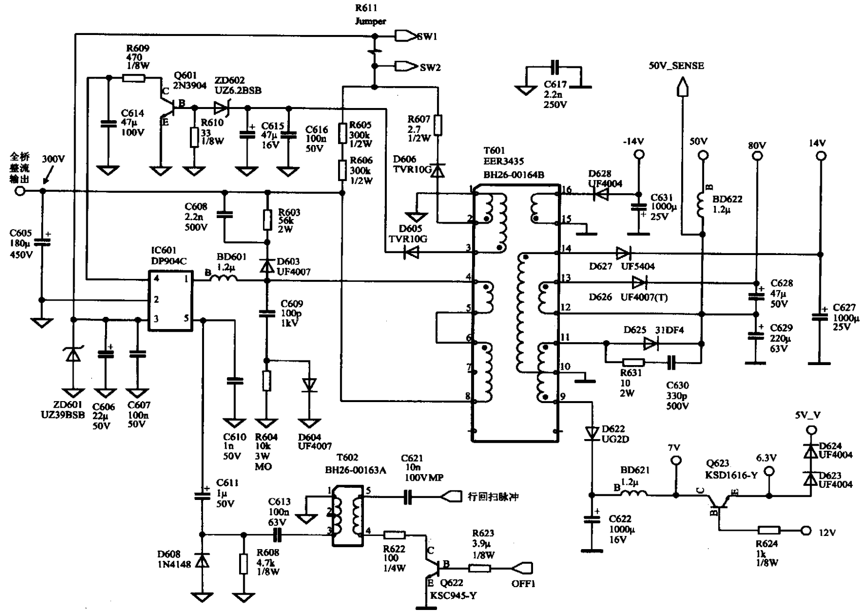
图 37 DP904C 典型应用电路
