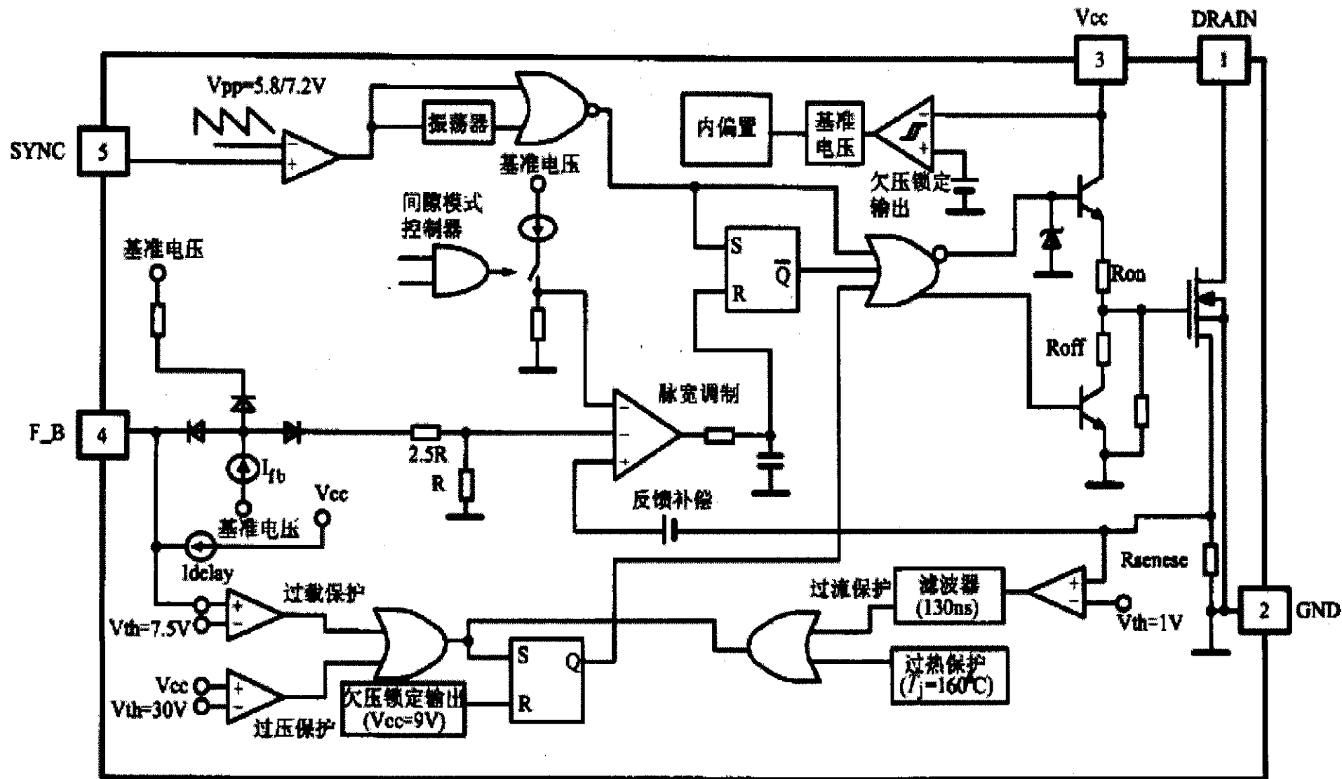
图 36 DP904C 内部等效图
