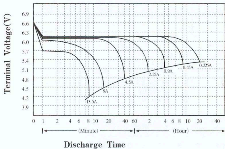
Характеристики разряда.
