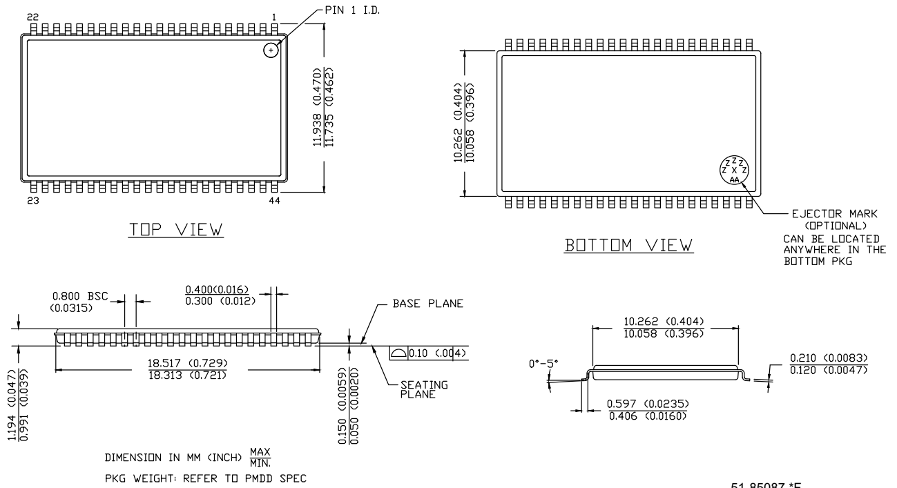
図 17. 44 ピン TSOP II パッケージ図、51-85087
