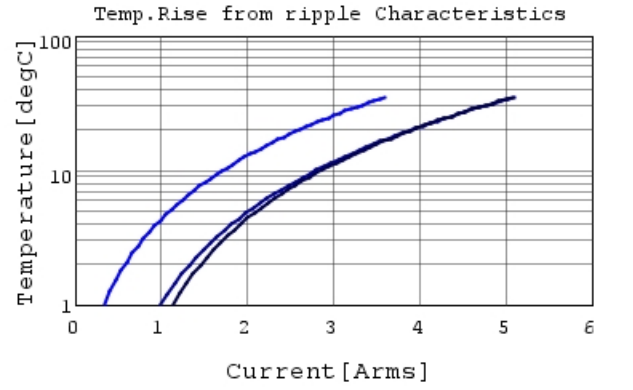
GRM188R60J106ME47 Temp.rise — 80kHz —
