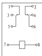
接线图
