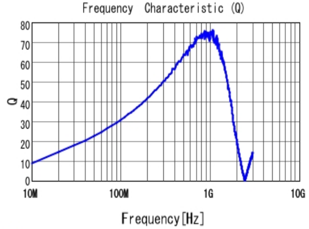
■ LQW18AN75NJ00 Q
