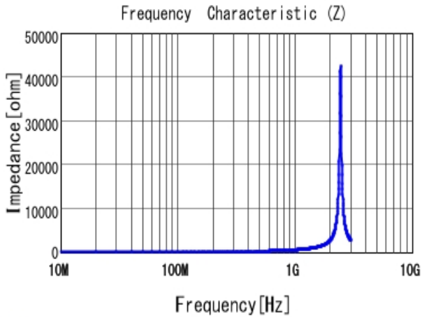
■ LQW18AN75NJ00 |Z|
