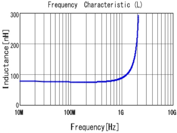
■ LQW18AN75NJ00 L
