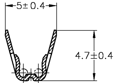
断面 B-B SECT B-B
