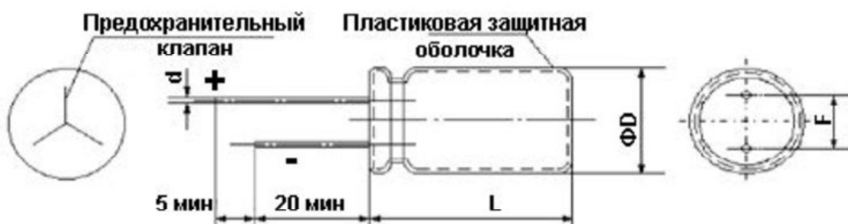
Габаритные размеры
