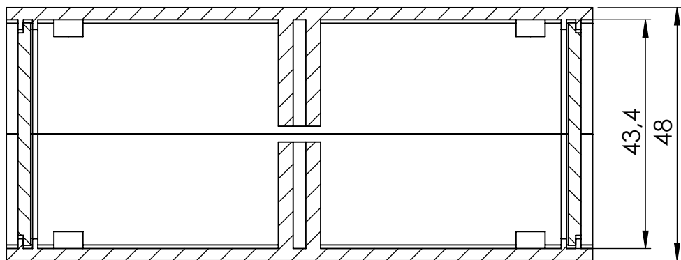
PRZEKRÓJ A-A
