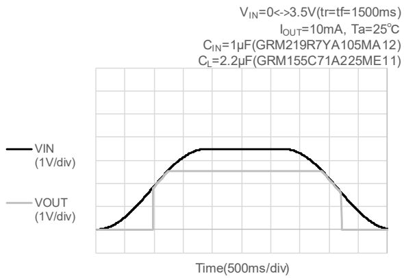
(10-1) V_{OUT(T)}=2.5V
