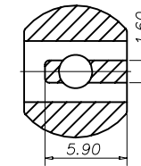
SECTION D-D
