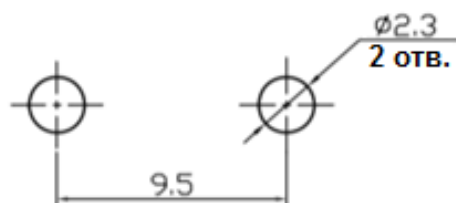
Отверстия для крепления
