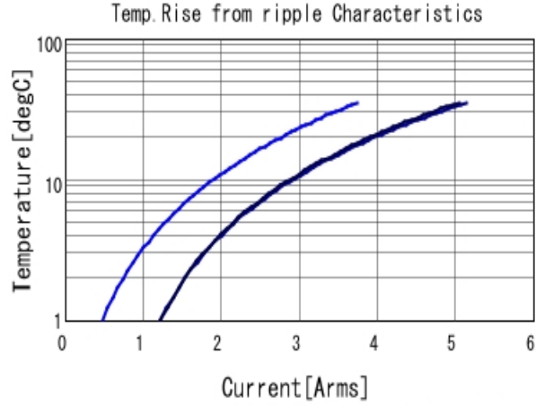
GRM188R60G106ME47 Temp. rise ■ 80kHz ■ 400kHz ■ 800kHz
