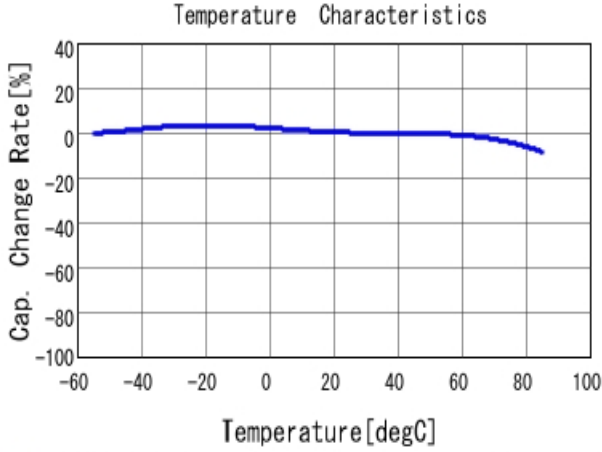
■ GRM188R60G106ME47 C-Temp. capchange, DCO. 0V, ACO. 5Vrm
