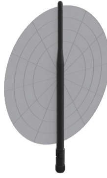
YZ-Plane Gain
