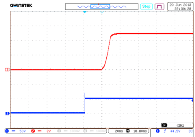
Рис. 25. Установление U_{\text{вых.ном}} с момента подачи U_{\text{вх.ном}} .
