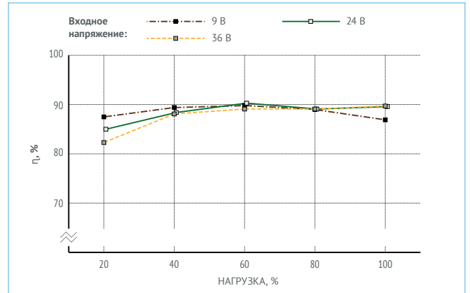
Рис. 9. VDRI30B12.
