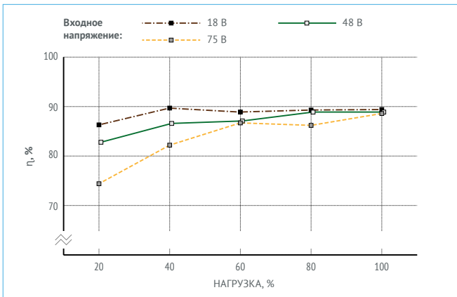
Рис. 17. VDRI30W24.
