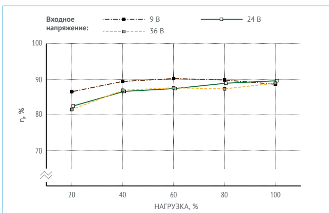
Рис. 8. VDRI30B09.
