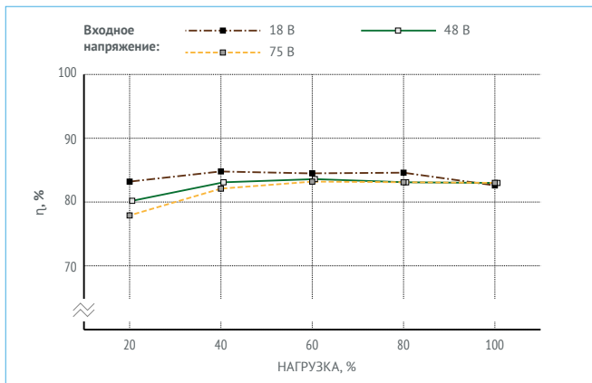
Рис. 13. VDRI30W3,3.
