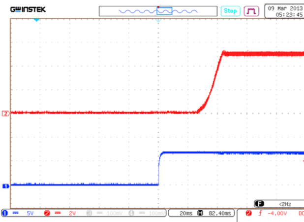
Рис. 19. Установление U_{\text{ВЫХ.НОМ}} с момента подачи ДУ (соединение выводов «ВКЛ» и «-ВХ»).
