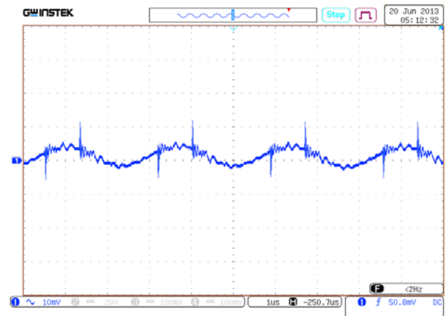
Рис. 26. Осциллограмма пульсаций U_{\text{вых.ном}} .
