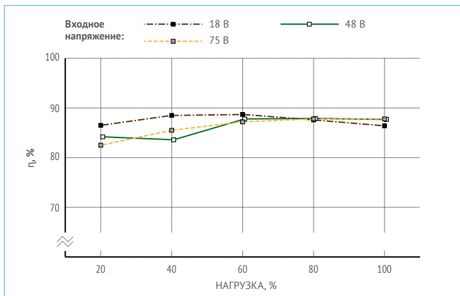
Рис. 14. VDRI30W05.
