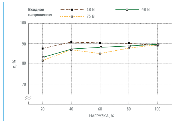
Рис. 15. VDRI30W09.
