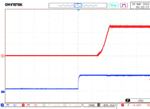
Рис. 20. Установление U_{\text{ВЫХ.НОМ}} с момента подачи ДУ (управляющий сигнал).
