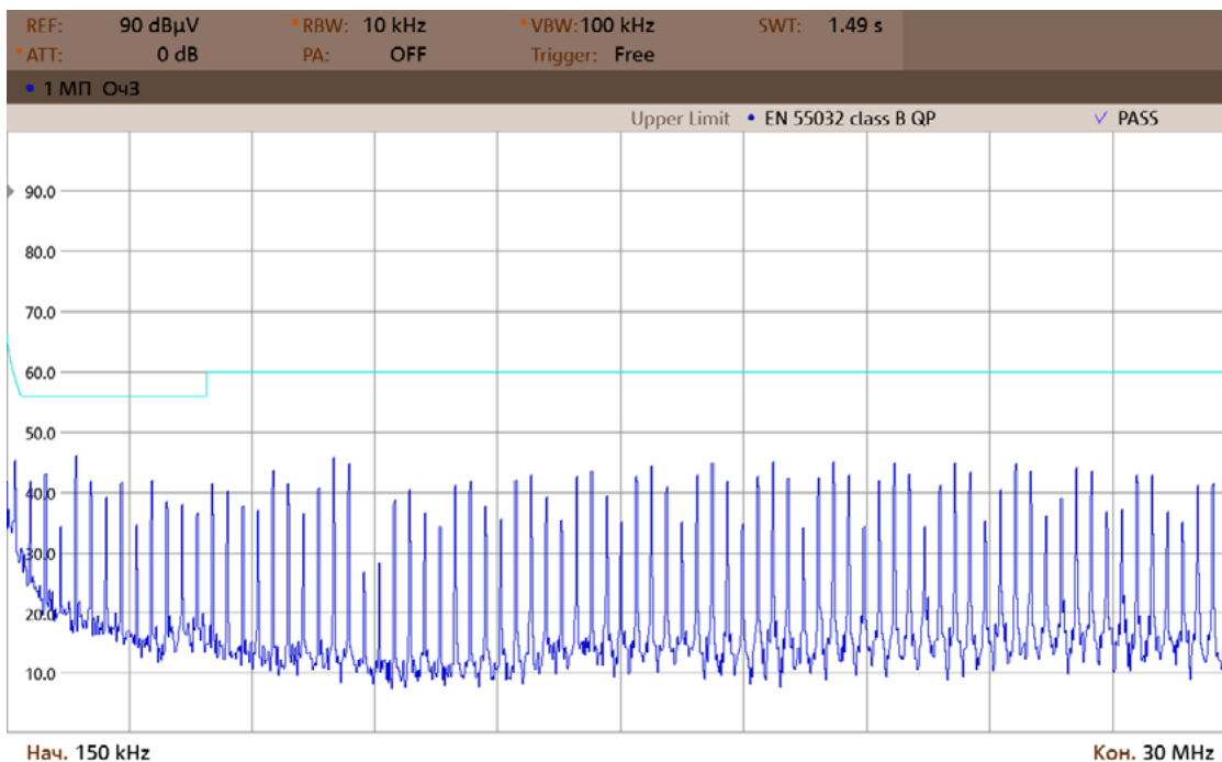
Рис. 34. Спектрограмма соответствия EN55032 Class B (0,15–30 MHz).
