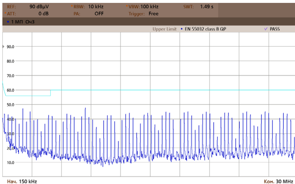
Рис. 28. Спектрограмма соответствия EN55032 Class B (0,15–30 MHz).
