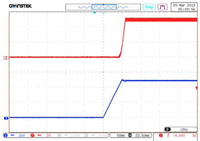
Рис. 21. Установление U_{\text{ВЫХ.НОМ}} с момента подачи U_{\text{ВХ.НОМ}} .
