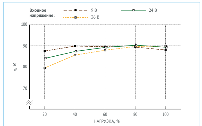
Рис. 10. VDRI30B15.
