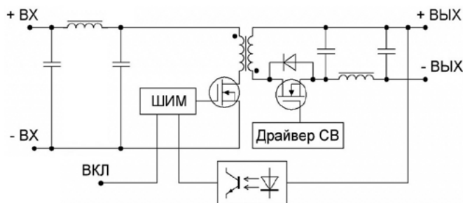
Рис. 1. Топология VDRI20, VDRI30.
