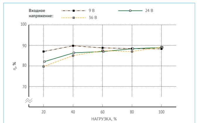
Рис. 11. VDRI30B24.
