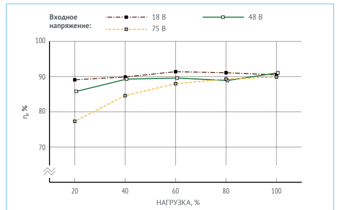
Рис. 16. VDRI30W15.
