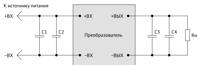
Рис. 2. Схема включения VDRI20, VDRI30.
