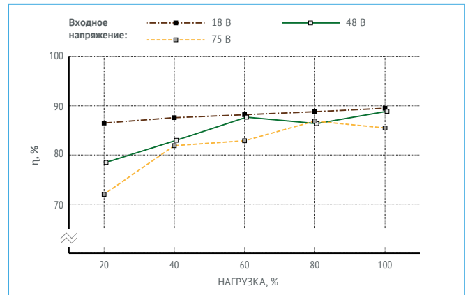
Рис. 18. VDRI30W48.
