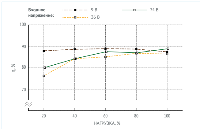
Рис. 12. VDRI30B48.
