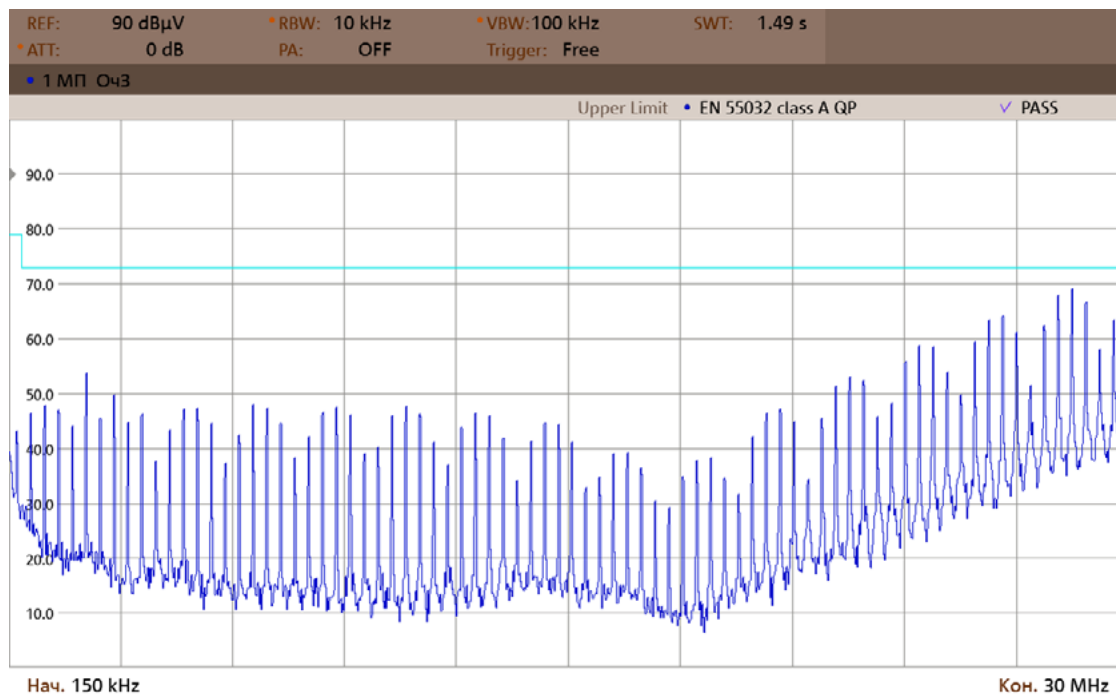
Рис. 27. Спектрограмма соответствия EN55032 Class A (0,15–30 MHz).
