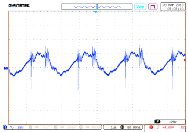
Рис. 22. Осциллограмма пульсаций U_{\text{ВЫХ.НОМ}} .
