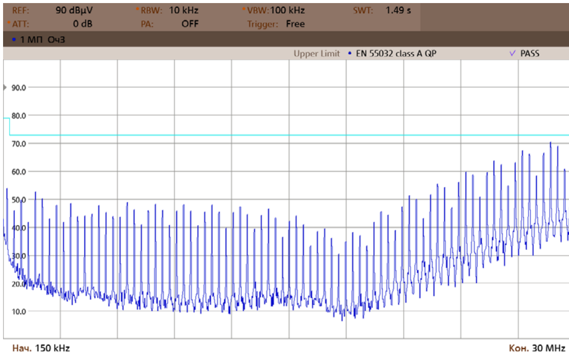
Рис. 33. Спектрограмма соответствия EN55032 Class A (0,15–30 MHz).
