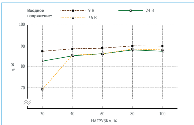
Рис. 7. VDRI30B05.
