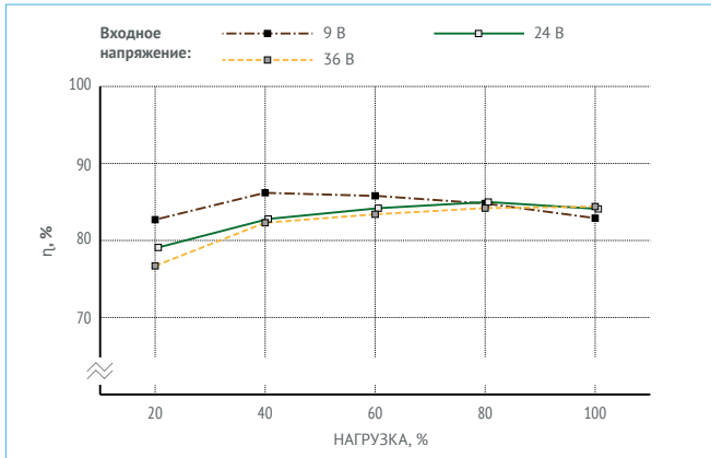
Рис. 6. VDRI30B3,3.
