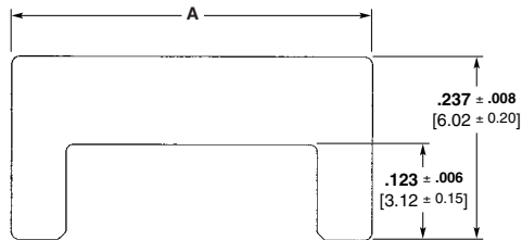
Feed-Thru
