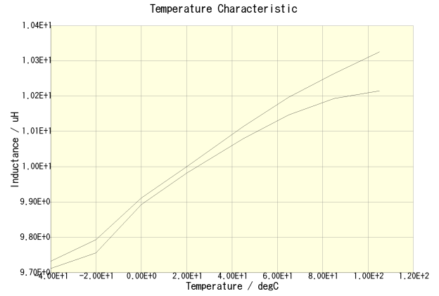
VLCF4028T-100M1R0-2(DC = 0A) VLCF4028T-100M1R0-2(DC = 0.53A)
