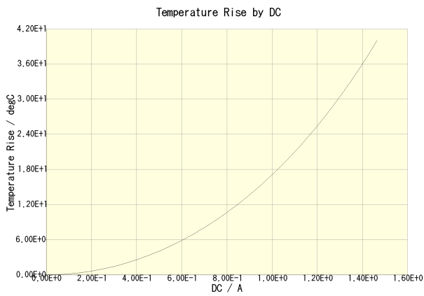
VLCF4028T-100M1R0-2(Amb. Temp. = 20degc)
