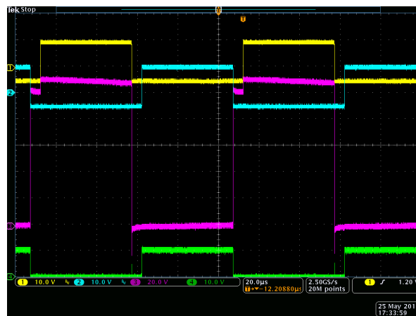
C_L=1\text{ nF}
