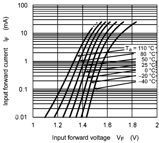
Fig. 13.2.1 I_F - V_F
