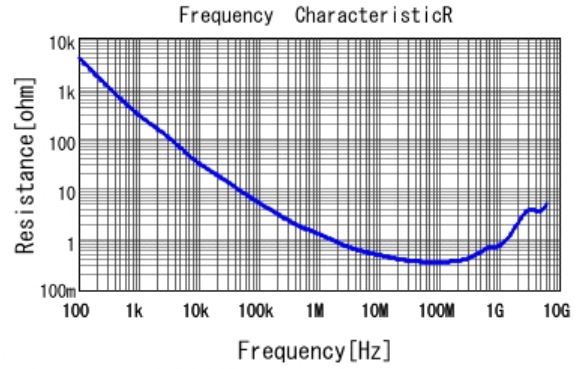
■ GCJ188R71H222KA01 R DCOV, 25degC
