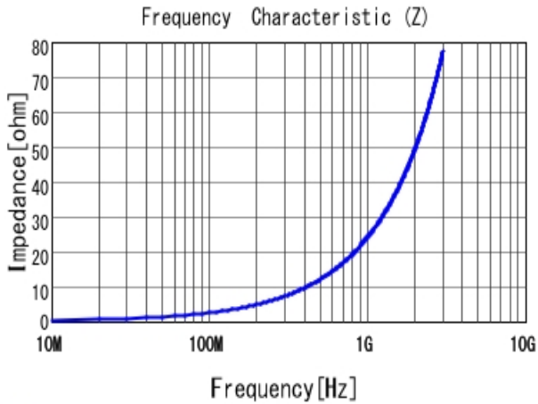
■ LQW15AN3N9D00 |Z|
