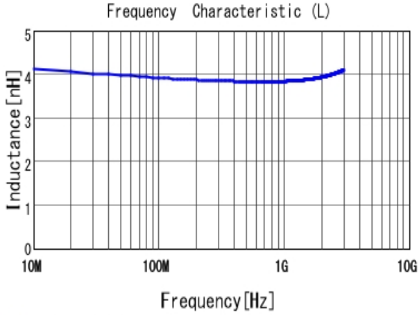
■ LQW15AN3N9D00 L
