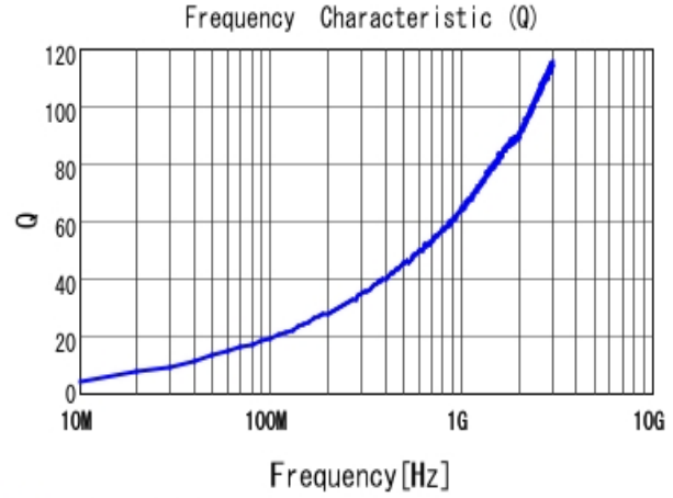
■ LQW15AN3N9D00 Q
