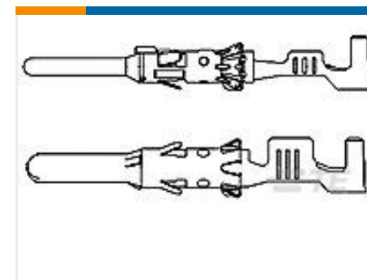
TE Part # 1-962972-0 2,5MM STIFTKONT EDS
