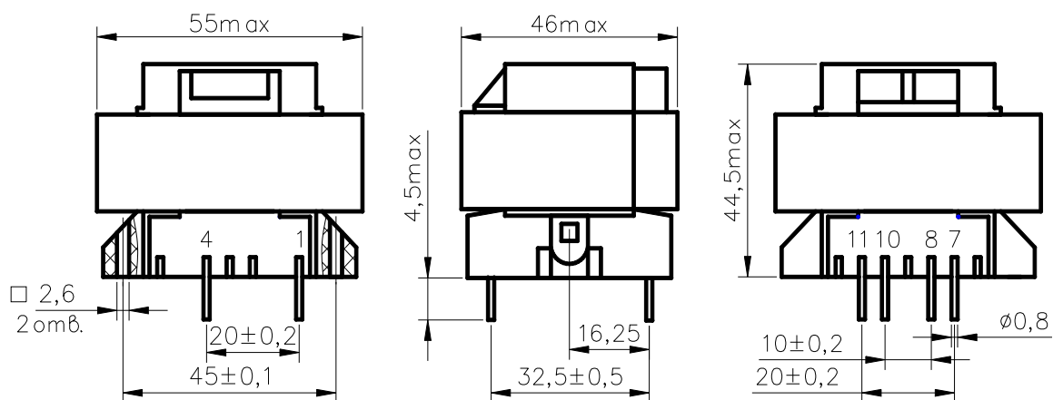
Общий вид трансформатора
