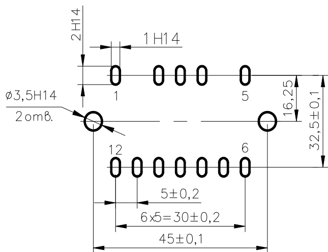
Рекомендуемая разметка для крепления
