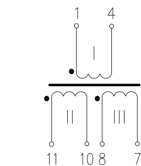
Схема электрическая
