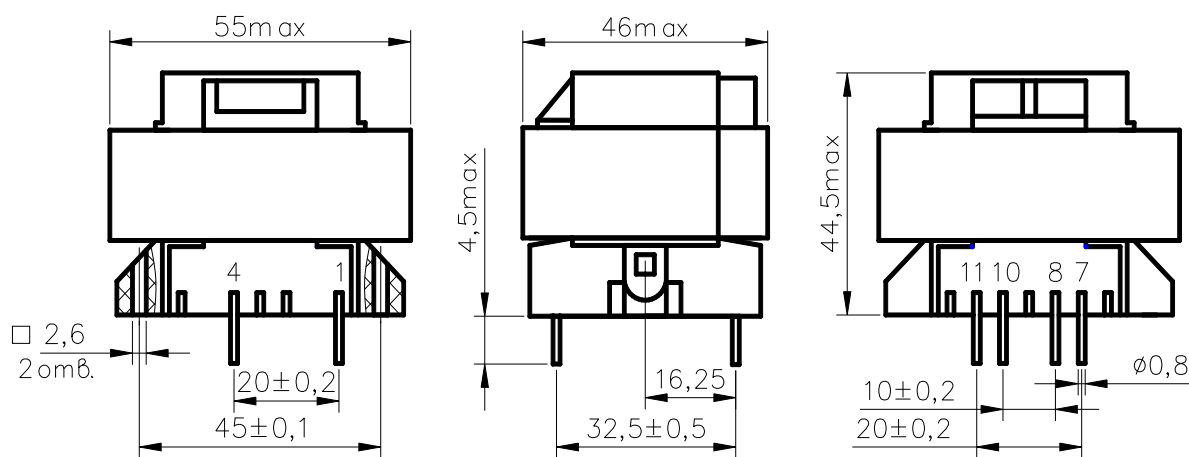
Общий вид трансформатора
