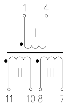
Схема электрическая
