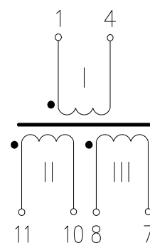
Схема электрическая
