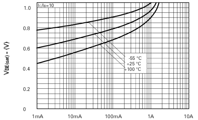
I C -Collector Current V BE(sat) v I C
