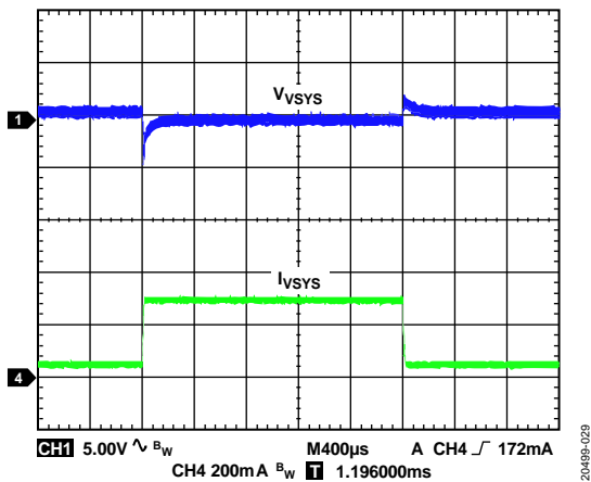
Figure 28. V_{SYS} Load Transient, I_{VSYS} = 50\text{ mA} to 300\text{ mA}
