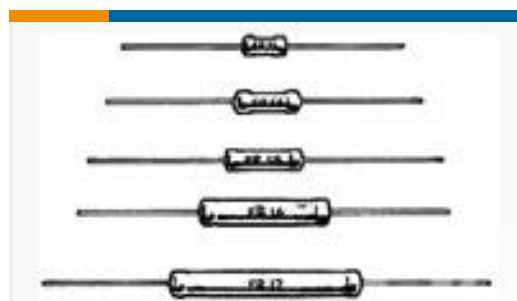
TE Part #1-1623746-6 ER74 1R8 5% AMMO PK
