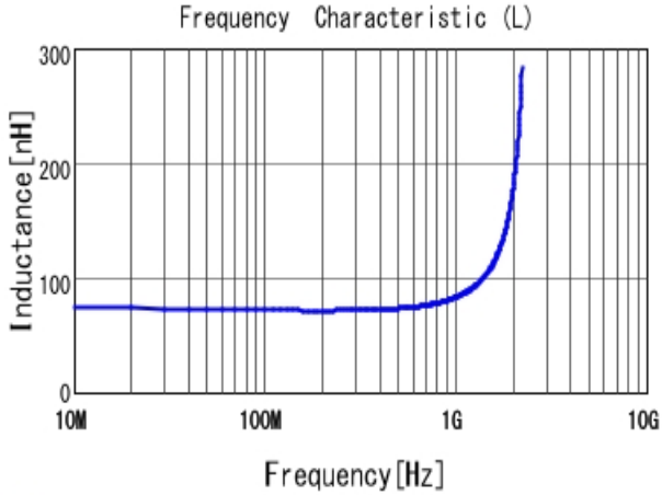
■ LQW18AN72NG00 L
