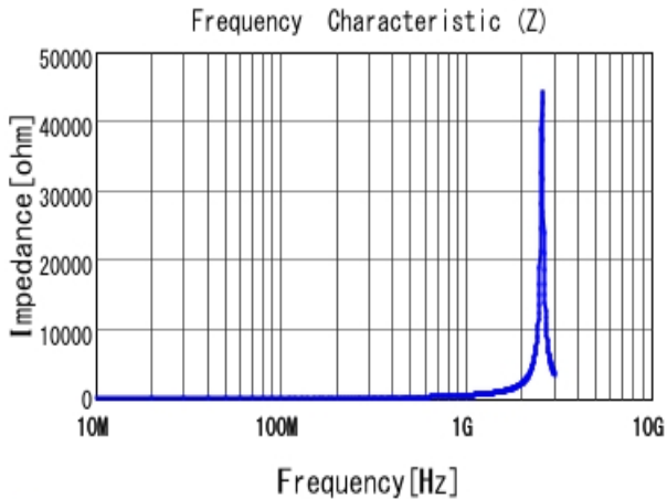
■ LQW18AN72NG00 |Z|
