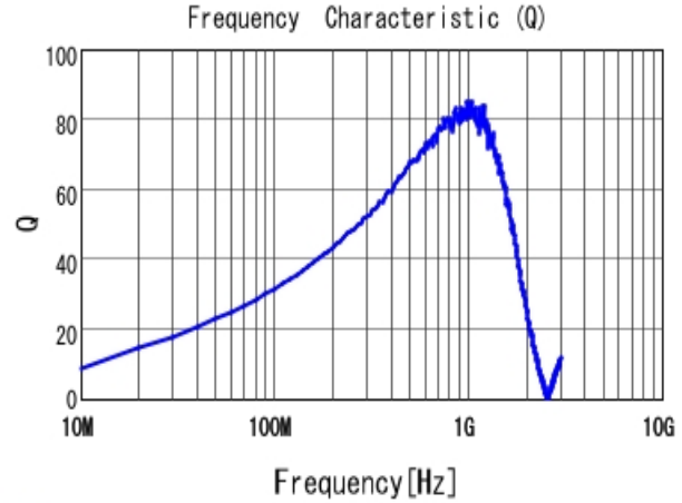
■ LQW18AN72NG00 Q
