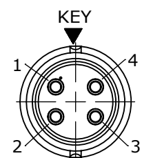
WIRING END W6280-4SG-P-3XX
